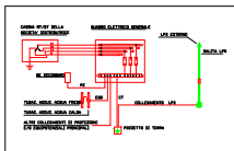
PARTICOLARE NERZA A TERRA E COLLEGAMENTO SOSPENSIONE
