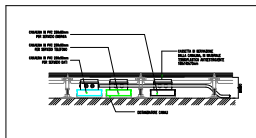
PARTICOLARE CASSETTA DI SOSPENSIONE SOTTOPAVIMENTO
